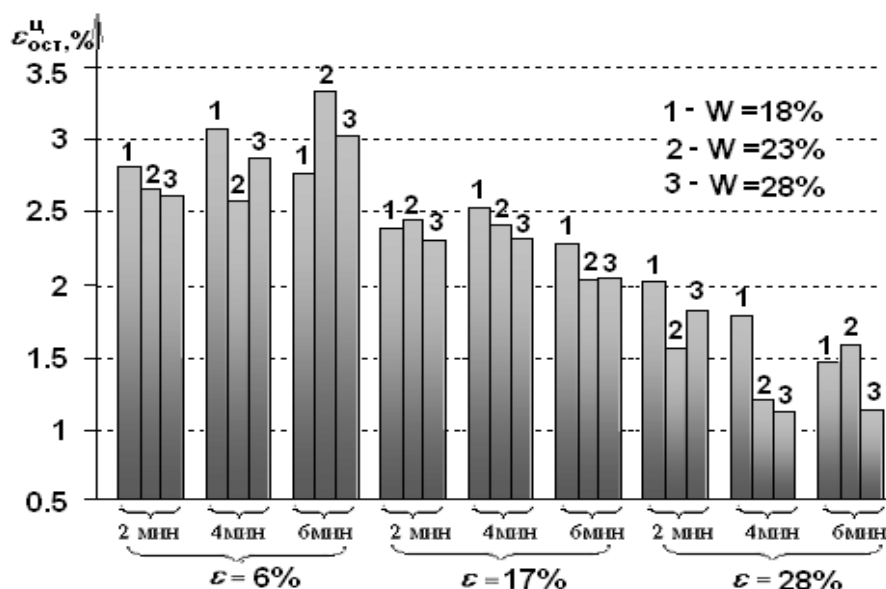
Рисунок 3 – Остаточная циклическая деформация систем материалов: а – кожа «Софт» + термобязь + трикотаж; б – кожа «Софт» + нетканый материал + трикотаж
