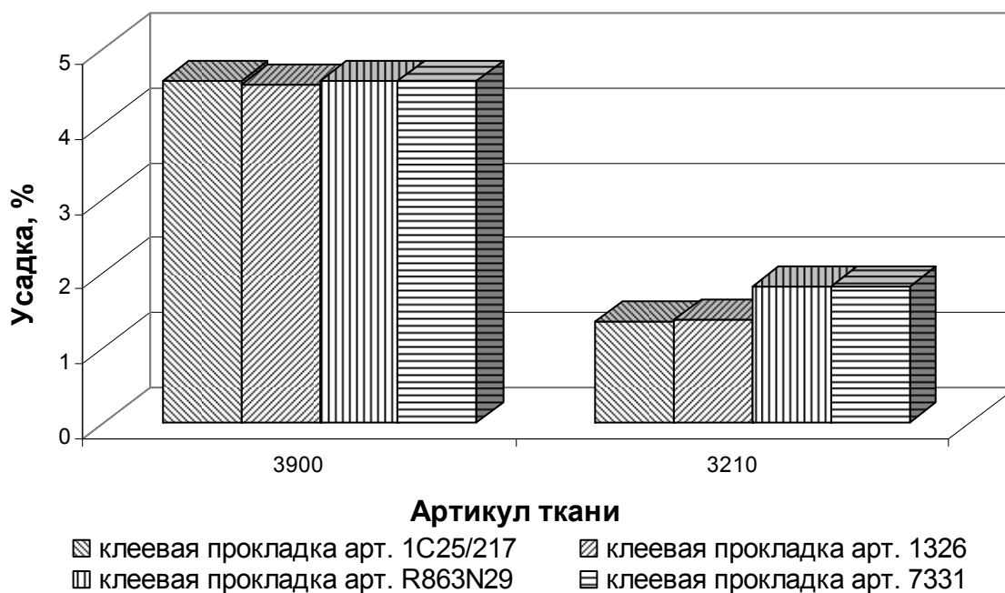
Рисунок 3 – Зависимость усадки клеевого пакета после дублирования от степени растяжимости эластичных костюмных тканей
