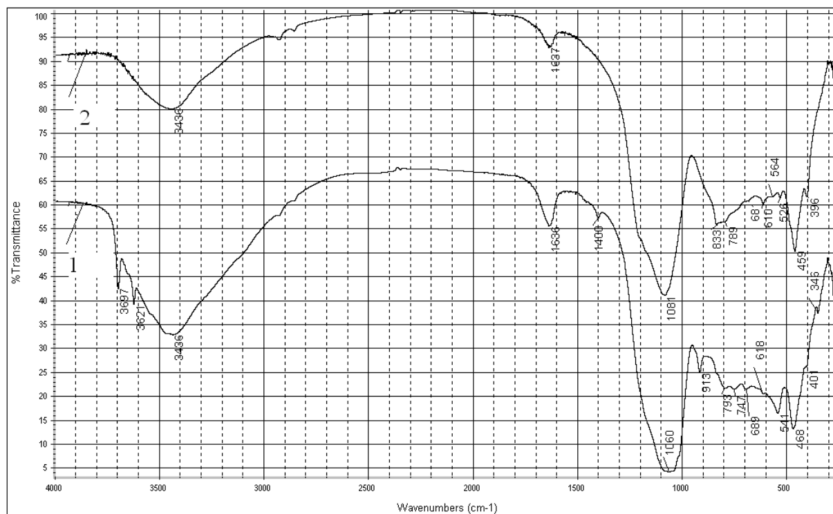
Рисунок 1 – ИК-спектр исходного (1) и отработанного (2) катализатора крекинга
