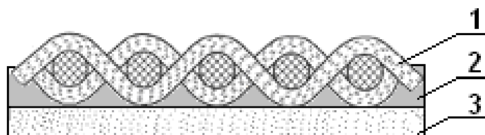
Рисунок 1 – Клеевое соединение составляющих текстильного настенного покрытия: 1 – тканое полотно; 2 – клей; 3 – полотно основы
