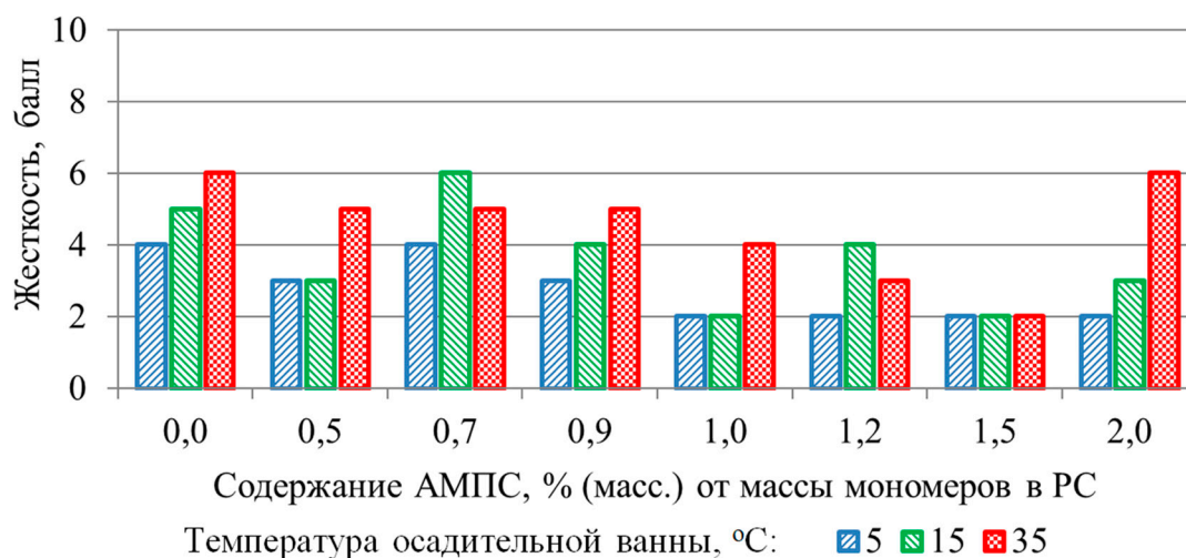
Рисунок 9 – Влияние содержания АМПС в реакционной смеси и температуры осадительной ванны на жесткость волокон на основе поли[АН-со-МА-со-АМПС] (65%-ный водный раствор ДМФ)
