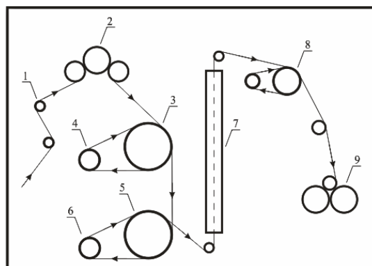
Рисунок 2 – Схема стэнда ОСВ-1:
