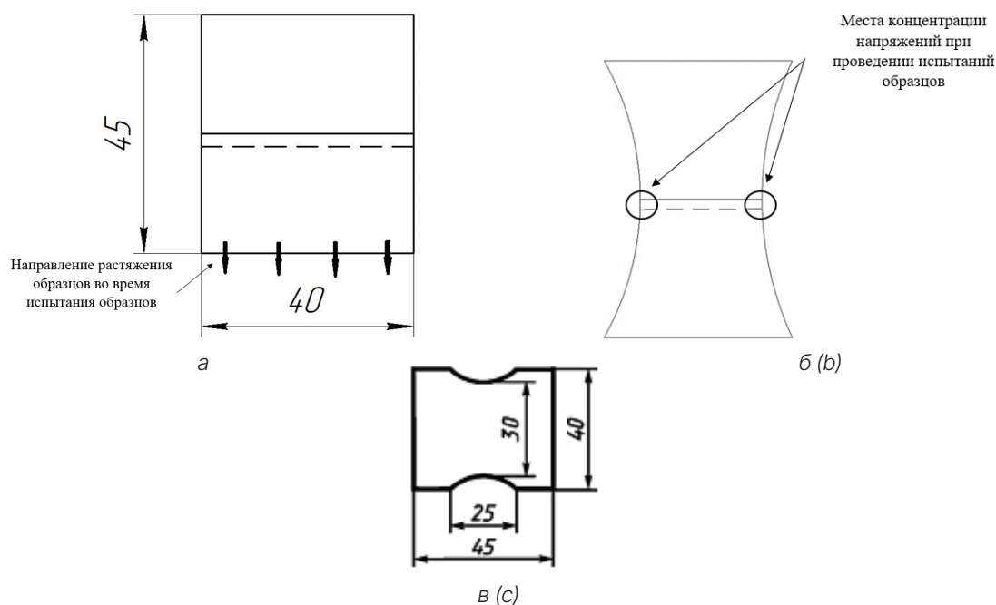
Рисунок 2 – Формы образцов для испытаний ниточных соединений по ГОСТ 9290:
