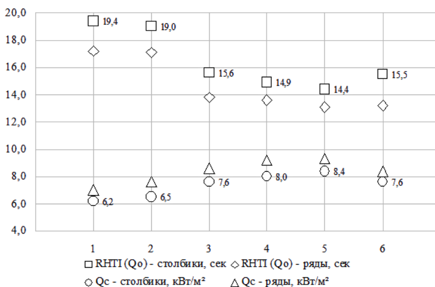
Рисунок 3 – Индекс передачи теплового излучения RHTI(Q_o) и плотность пропущенного теплового потока Q_c при плотности падающего теплового потока Q_o равной 20 \text{ кВт/м}^2 для груза предварительного натяжения 40 грамм Figure 3 – Radiant Heat Transfer Index RHTI(Q_o) and transmitted heat flux density Q_c at incident heat flux density Q_o equal to 20 \text{ кВт/м}^2 for a pre-tensioned load of 40 grams
