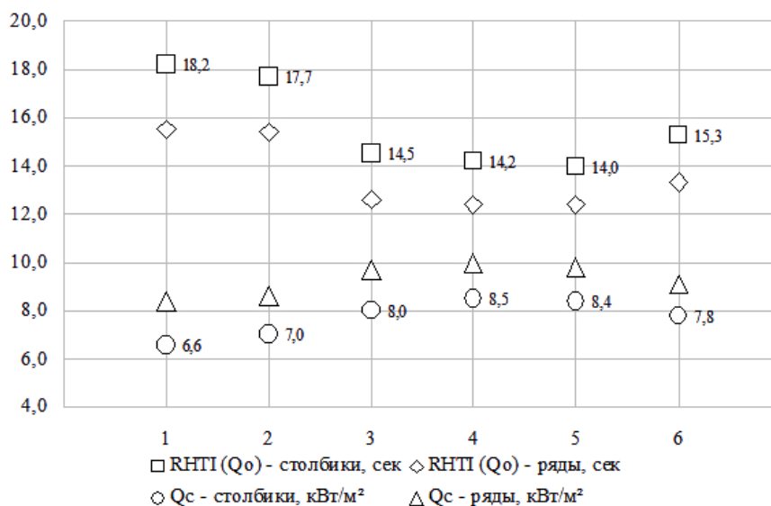
Рисунок 2 – Индекс передачи теплового излучения RHTI(Q_o) и плотность пропущенного теплового потока Q_c при плотности падающего теплового потока Q_o равной 20 \text{ кВт/м}^2 для груза предварительного натяжения 100 грамм Figure 2 – Radiant Heat Transfer Index RHTI(Q_o) and transmitted heat flux density Q_c at incident heat flux density Q_o equal to 20 \text{ кВт/м}^2 for a pre-tensioned load of 100 grams
