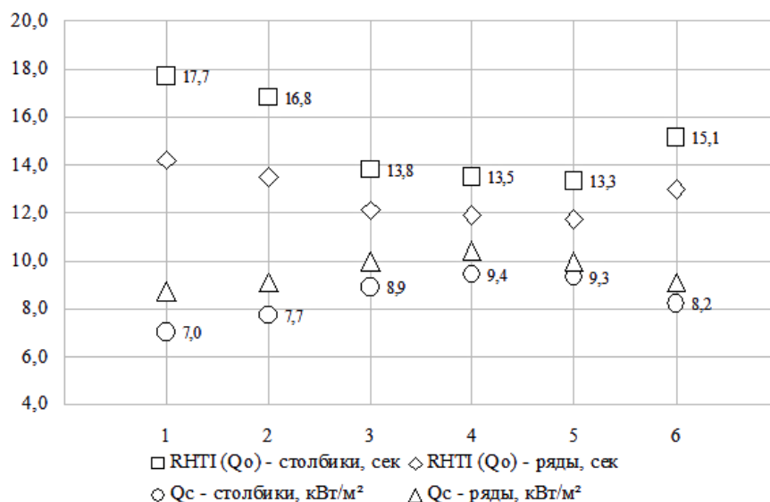
Рисунок 1 – Индекс передачи теплового излучения RHTI (Q_o) и плотность пропущенного теплового потока Q_c при плотности падающего теплового потока Q_o равной 20 кВт/м 2
